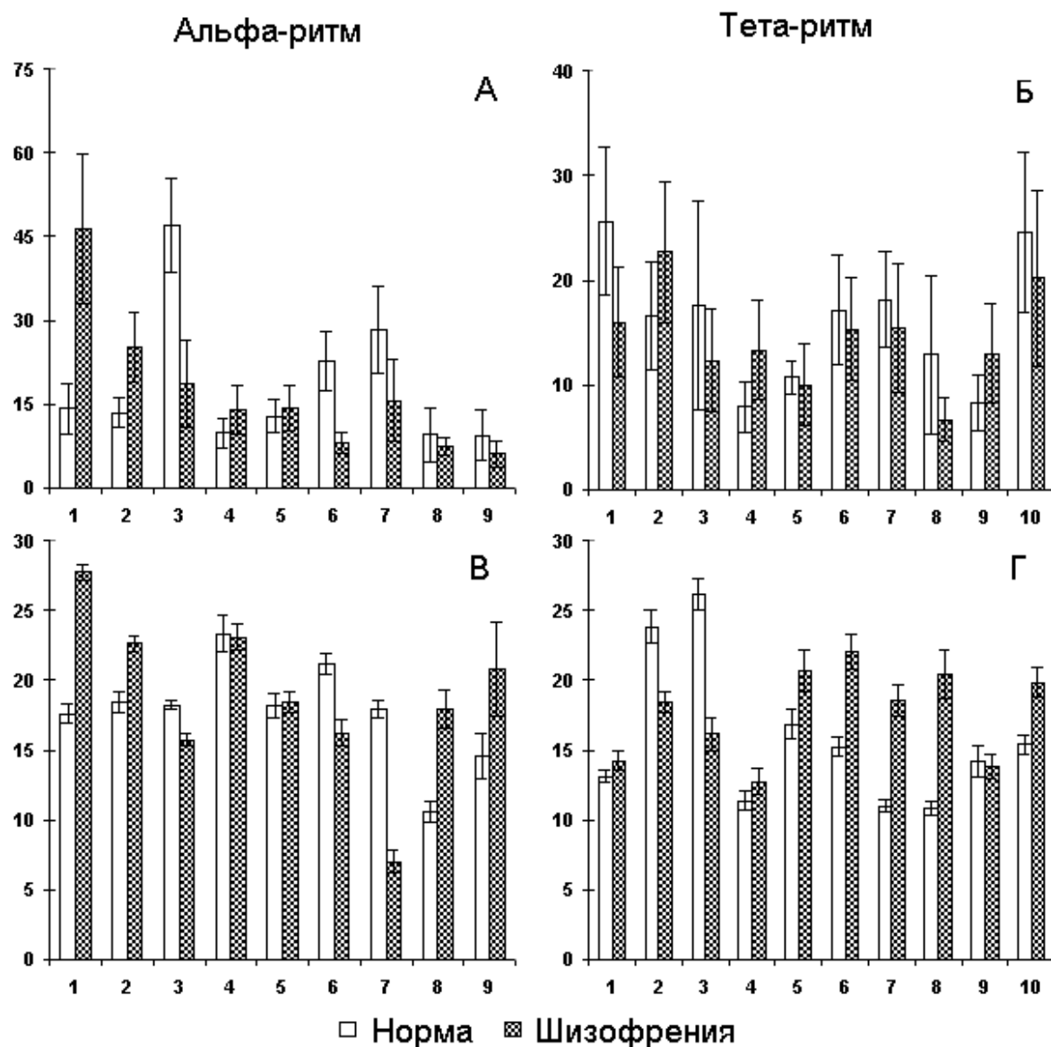
Рис. 4. Среднее число диполей (А,Б) и средний модуль дипольного момента (В,Г) в кластерах источников альфа-ритма (А,В) и тета-ритма (Б,Г). По оси абсцисс – среднее число диполей в кластере, по оси ординат номер кластера. Статистически достоверны различия в кластерах 1-3,6 ( p < 0.05 ) для среднего числа диполей альфа-ритма (А). Нет статистически достоверных различий для среднего числа диполей тета-ритма (Б). Статистически достоверные различия среднего модуля дипольного момента в кластерах 1-3,6-9 ( p < 0.05 ) для альфа-ритма (В). Статистически достоверные различия среднего модуля дипольного момента в кластерах 2,3,5-8,10 ( p < 0.05 ) для тета-ритма (Г).
