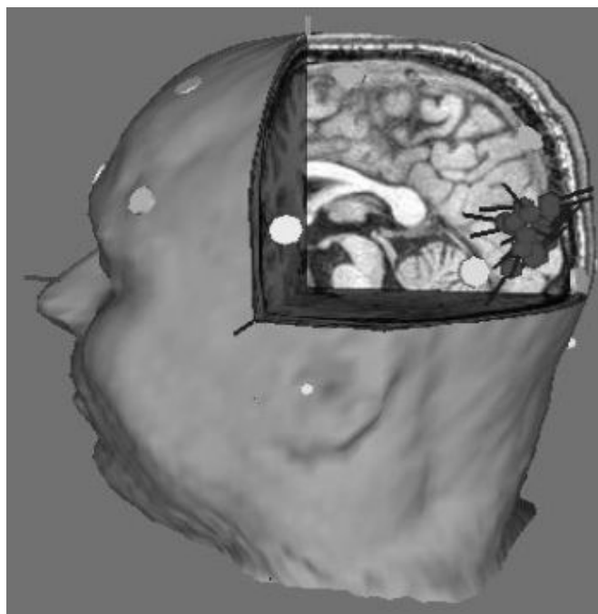
Рис. 1. Кластер диполей альфа - ритма в затылочной доле мозга. Крупные темные шарики - места локализации диполя, короткие отрезки – дипольный момент, диски –места расположения электродов ЭЭГ, светлые мелкие шарики – координатные метки.
