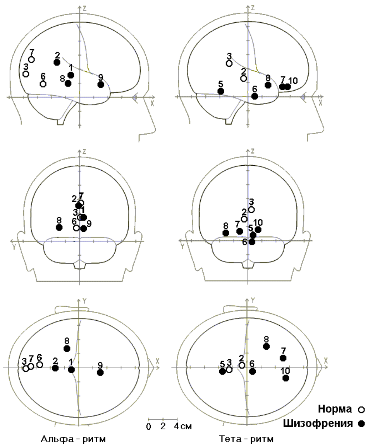
Рис. 3. Локализация дипольных кластеров для альфа- (слева) и тета-ритмов (справа) относительно контура мозга и головы. Оси X, Y, Z – пространственные координаты. Дипольные кластеры, достоверно различимые по локализации для альфа – ритма (кластеры 1-3,6; слева), а также по модулю дипольного момента для альфа-ритма (1-3,6-9; слева) и тета-ритма (кластеры 2,3,5-8,10; справа). Стандартное отклонение от центра кластера для источников альфа-ритма: 1-7-й кластеры от 1.3 до 1.7 см; 8-й кластер– 2.4 см и 9-й кластер– 3.0 см; для источников тета-ритма от 1.6 до 2.7 см.
