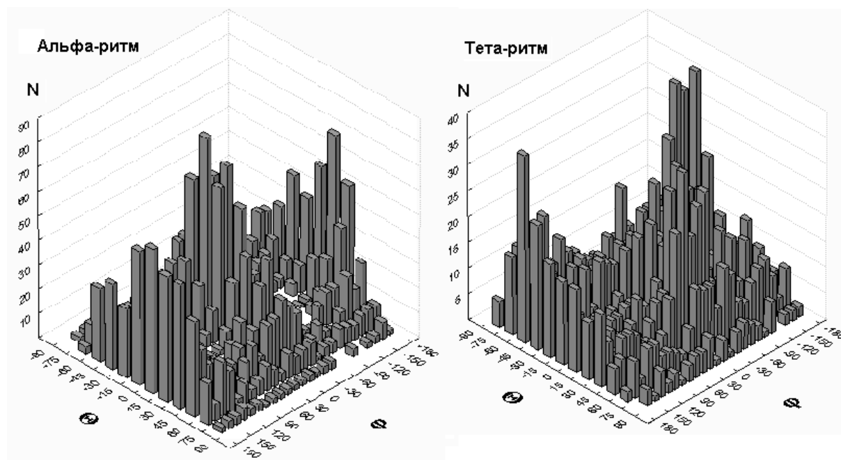
Рис.5 Распределение ориентаций дипольных моментов по углам \Theta и \varphi для локализованных источников альфа- и тета-ритма в идентифицированных кластерах. По осям: N – число диполей в кластере, \Theta и \varphi углы дипольных моментов. Преобладают направления с углами \Theta = 0 град. и \varphi = 0 град., 180 град., т.е. направления вдоль передне - задней оси головы.
